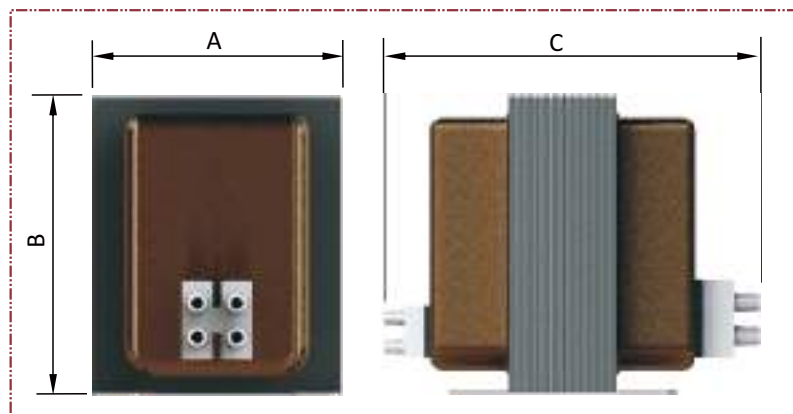
DIMENSIONAMENTO (mm)
