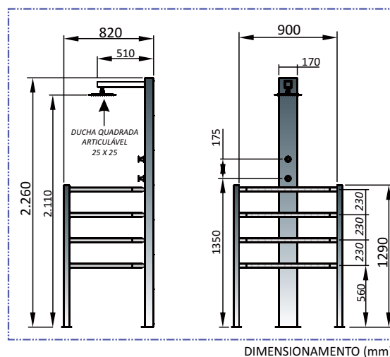
DIMENSIONAMENTO (mm)
