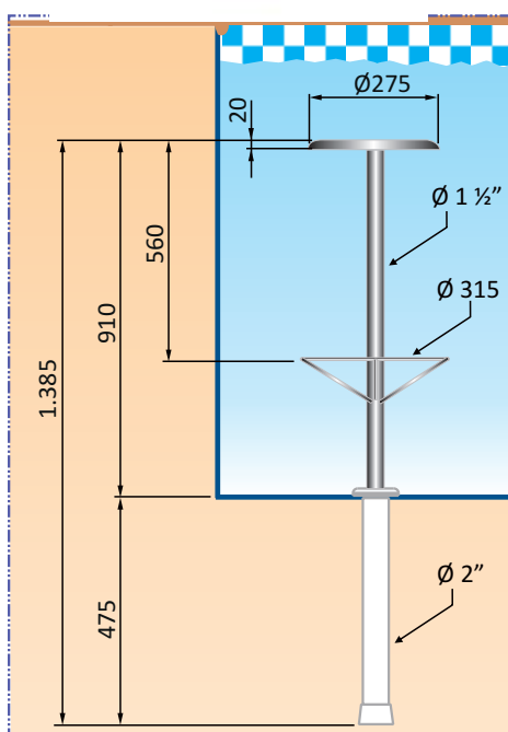
DIMENSIONAMENTO (mm)
