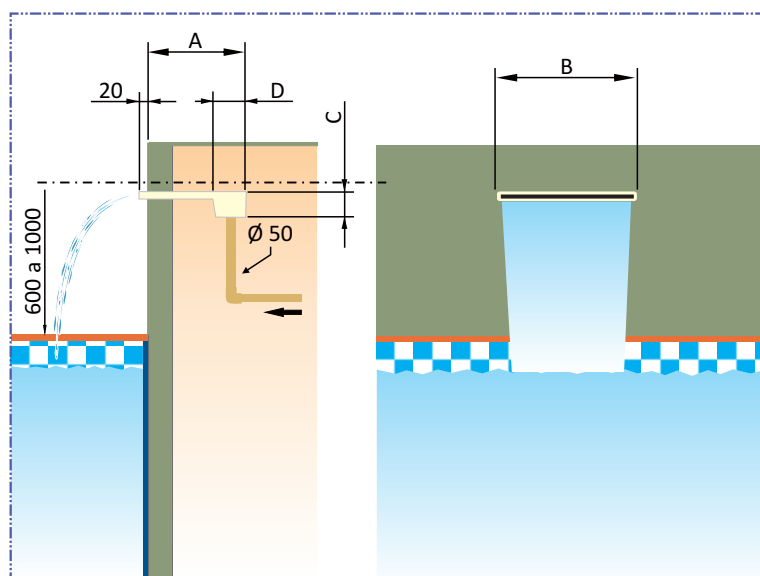
DIMENSIONAMENTO (mm)
