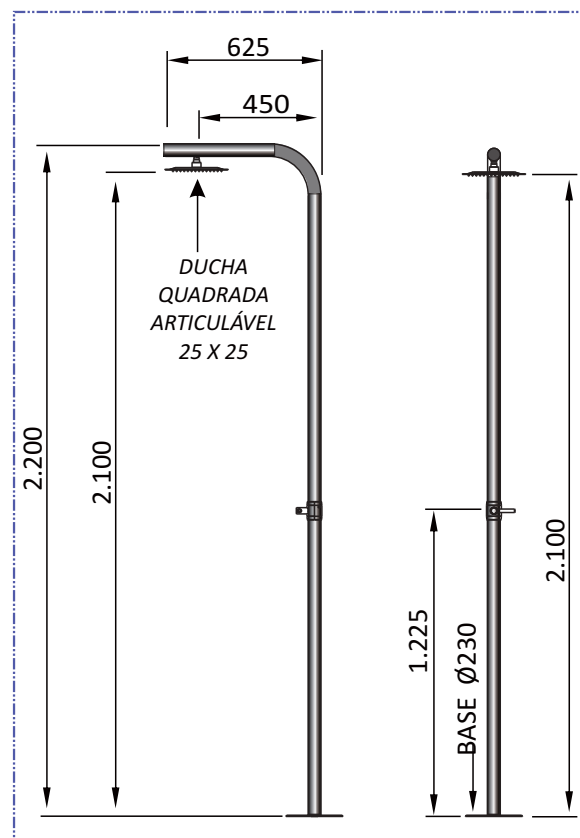
DIMENSIONAMENTO (mm)
