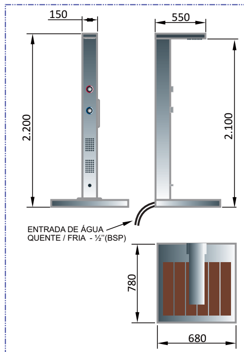
DIMENSIONAMENTO (mm)
