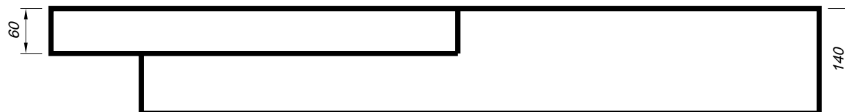
Corte AA
