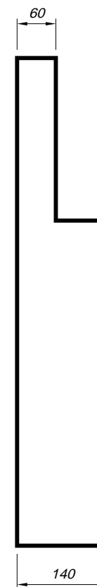
Corte BB
